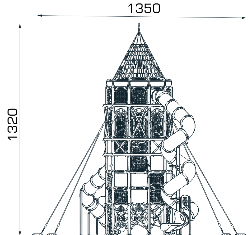
YAN GÖRÜNÜŞ / SIDE VIEW
