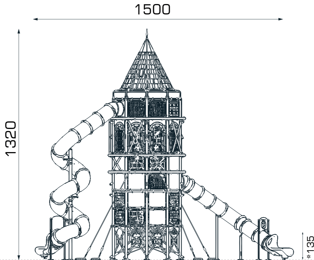
ÖN GÖRÜNÜŞ / FRONT VIEW
